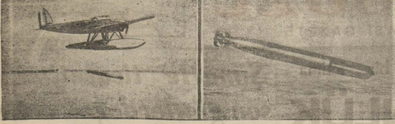
Bir torpil tayyaresi torpili atıyor
